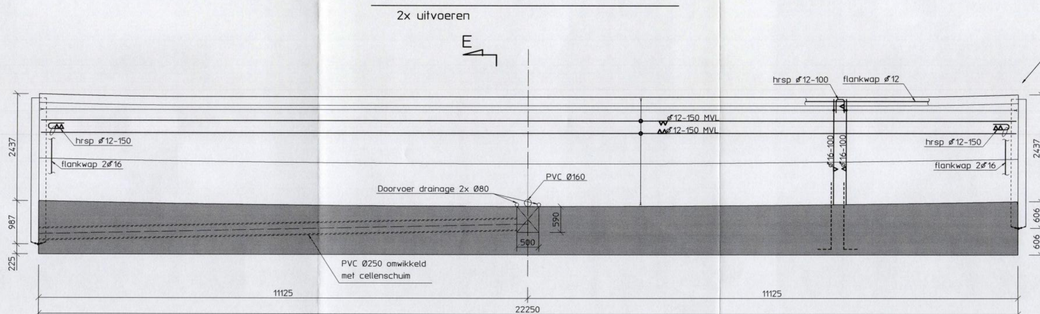
Doorsnede B
