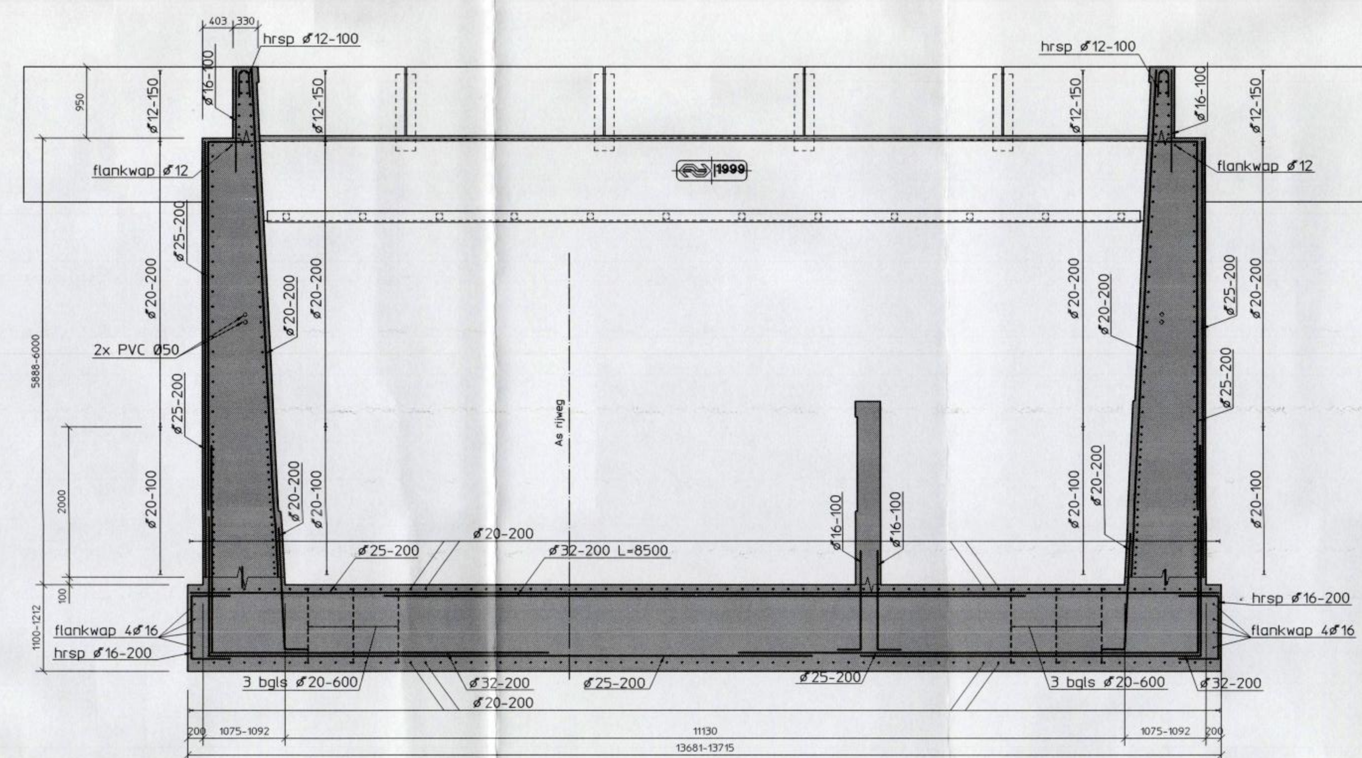
Doorsnede D
