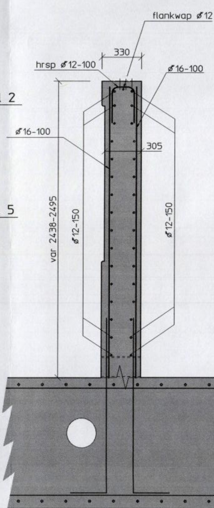
Doorsnede E
