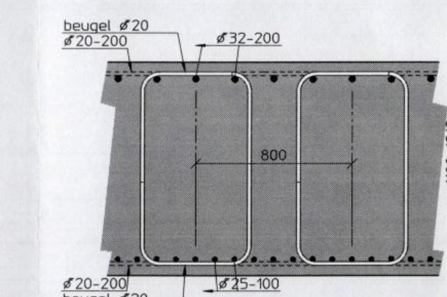
Beugels in vloer
