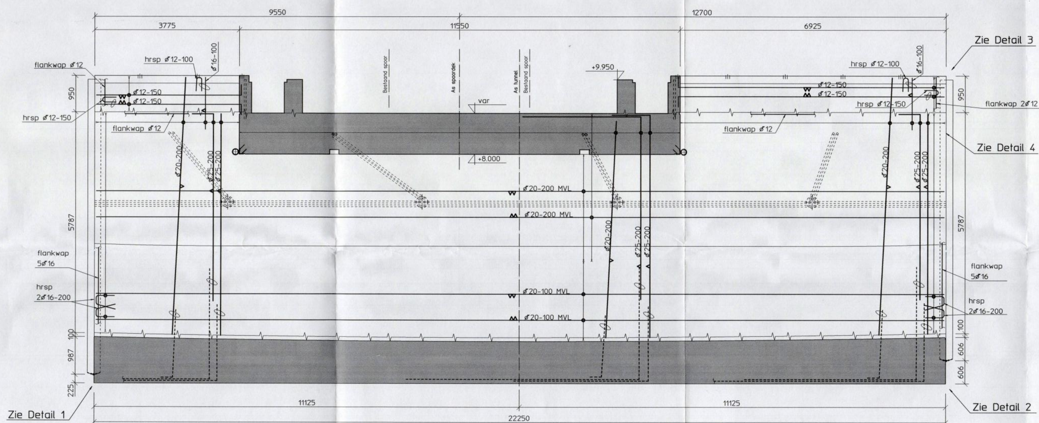
Doorsnede A
