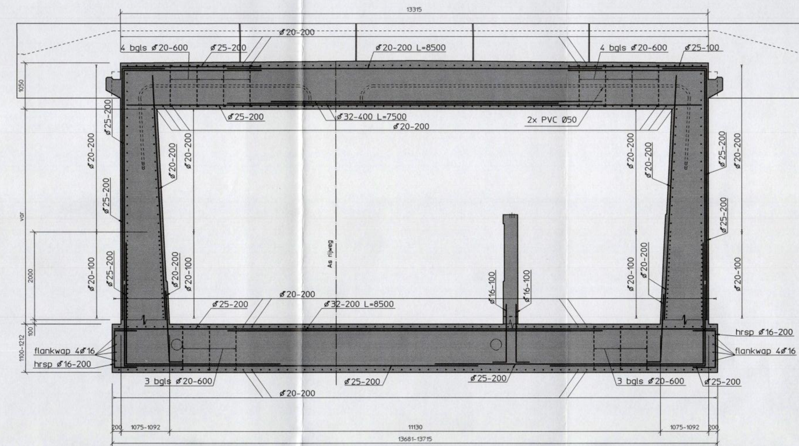
Doorsnede C
